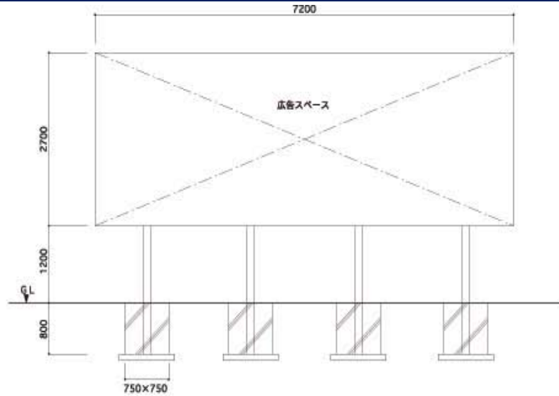
① 立面図 S=1/60
