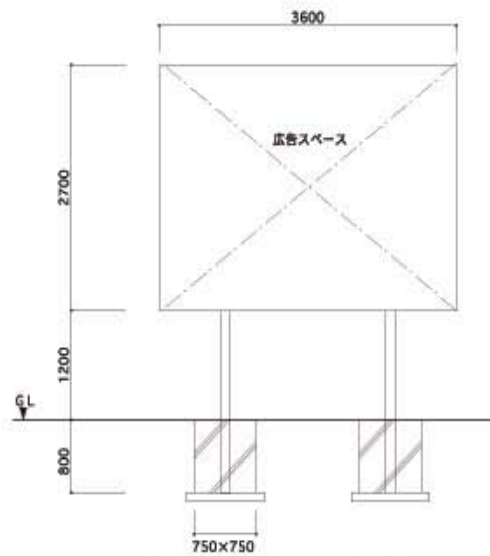
②～⑧ 立面図 S=1/60
